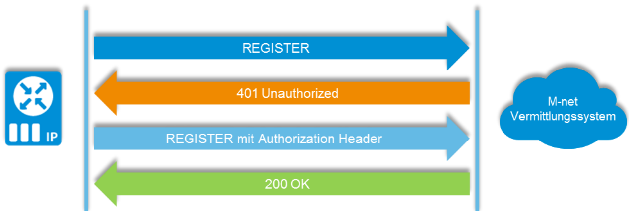
Abbildung 3: Beispiel Registrierungsablauf bei der Registrierung
