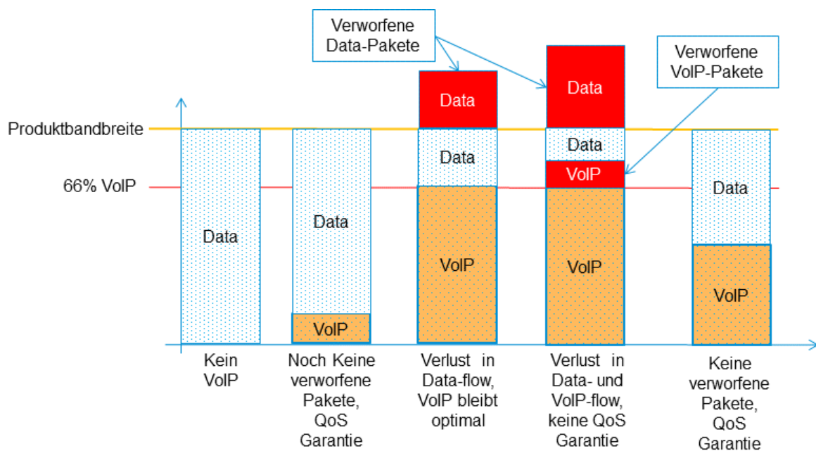
Abbildung 13: Szenarien mit bzw. ohne Verlust bei Daten-/VoIP-Strömen
