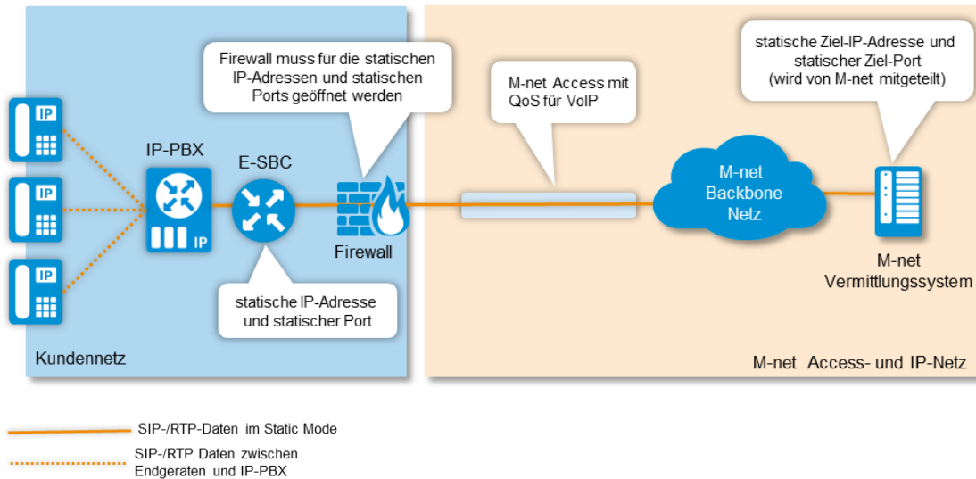
Abbildung 4: Beispiel Einfache Anschaltung einer IP-PBX im Premium SIP-Trunk Static Mode
