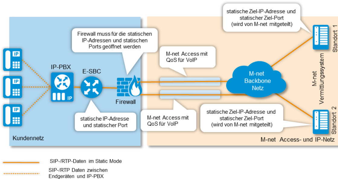
Abbildung 5: Anschaltung einer IP-PBX im Premium SIP-Trunk Static Mode und Loadbalancing
