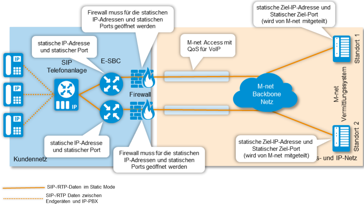
Abbildung 6: Anschaltung eines SIP-Trunk Accounts im Premium SIP-Trunk Static Mode mit Redundanz und Loadbalancing
