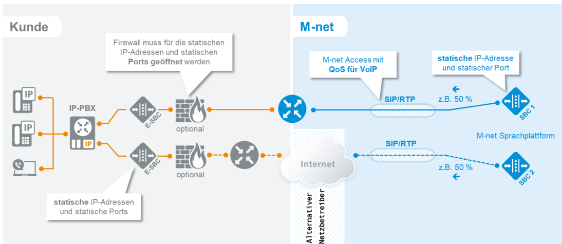
Abbildung 8: Anschaltung einer IP-PBX im SIP-Trunk Static Mode mit Redundanz und Loadbalancing über M-net Access (VoIP-Ready oder VoIP-Only) und Internet-Access durch Alternativenanbieter
