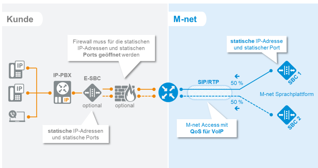
Abbildung 4: Anschaltung einer IP-PBX im SIP-Trunk Static Mode und Loadbalancing über M-net Access (VoIP-Ready oder VoIP-Only)
