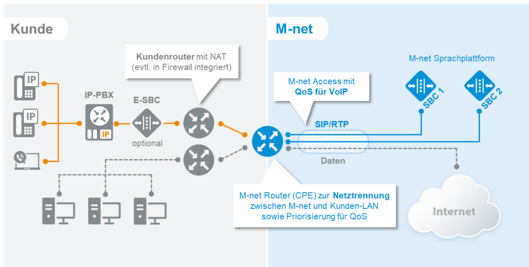
Abbildung 16: Beispiel Anschaltung der IP-PBX an die M-net Infrastruktur mit Verwendung eines Kundenrouters
