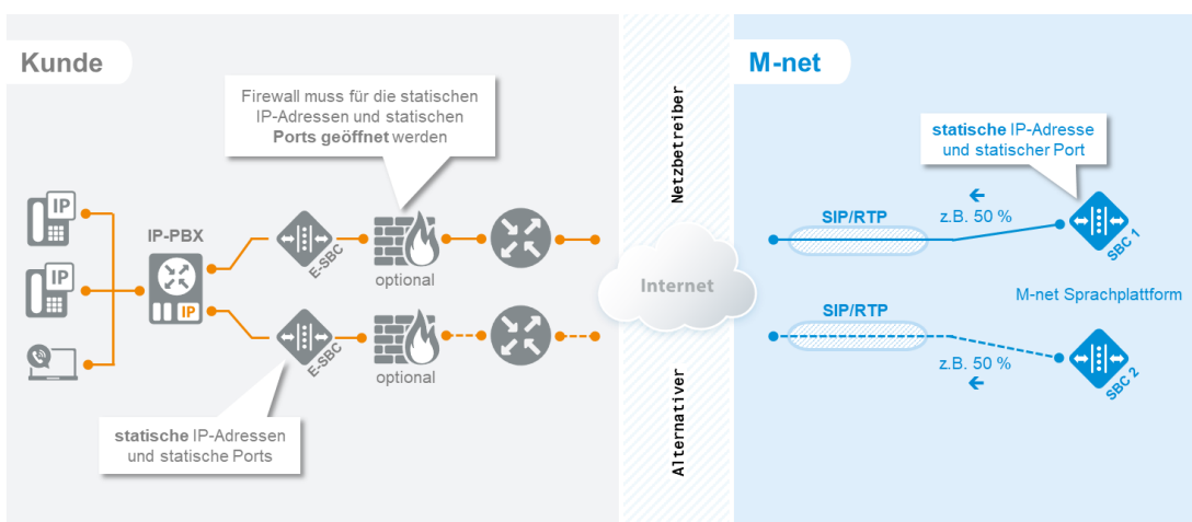
Abbildung 7: Anschaltung einer IP-PBX im SIP-Trunk Static Mode mit Redundanz und Loadbalancing über Internet-Access durch Alternativanbieter
