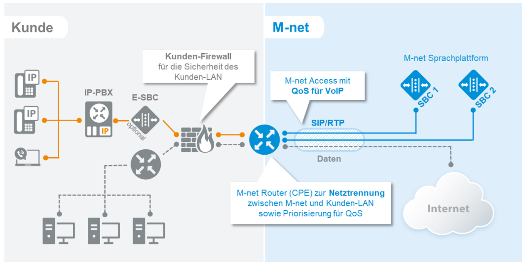
Abbildung 17: Beispiel Anschaltung der IP-PBX an die M-net Infrastruktur mit Verwendung einer Kunden-Firewall.
