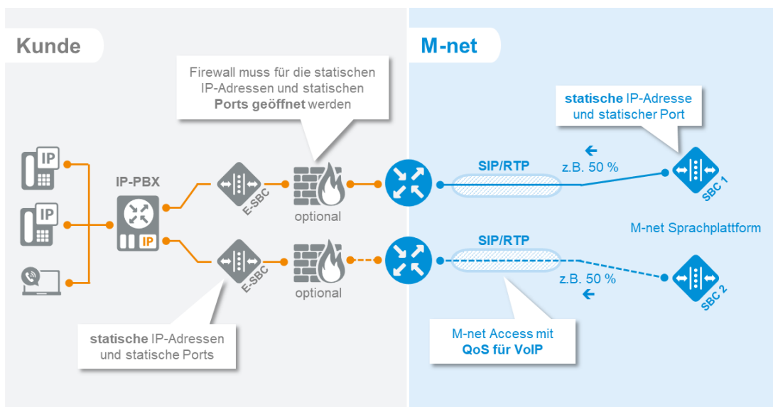
Abbildung 6: Anschaltung einer IP-PBX im SIP-Trunk Static Mode mit Redundanz und Loadbalancing über M-net Access (VoIP-Ready oder VoIP-Only)
