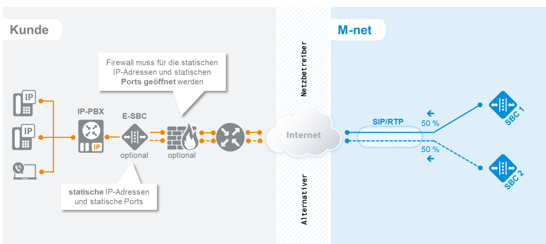
Abbildung 5: Anschaltung einer IP-PBX im SIP-Trunk Static Mode und Loadbalancing über Internet-Access durch Alternativenanbieter
