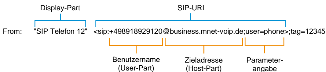
Beispiel und Aufbau eines Header Field (hier FROM-Header) in einer INVITE-Nachricht
