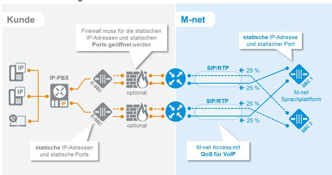
Abbildung 9: Anschaltung einer IP-PBX im SIP-Trunk Static Mode mit Redundanz und Loadbalancing bei Vollvermaschung über M-net Access (VoIP-Ready oder VoIP-Only)
