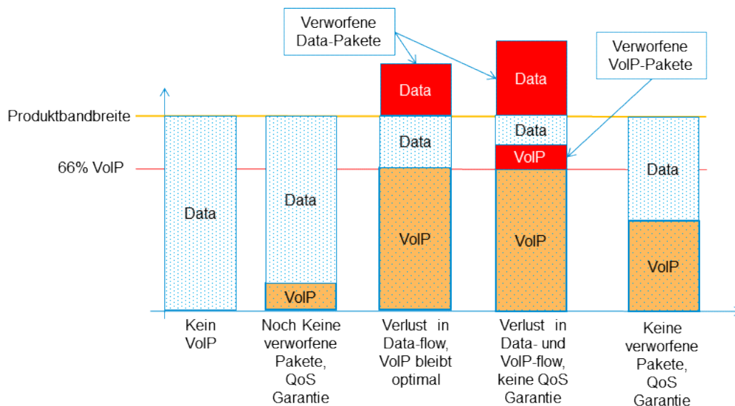
Abbildung 18: Szenarien mit bzw. ohne Verlust bei Daten-/VoIP-Strömen
