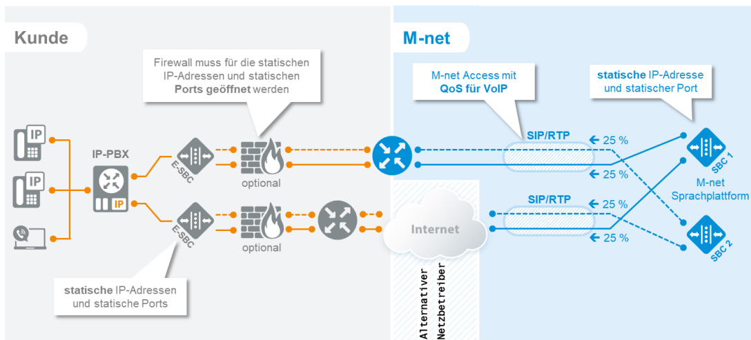
Abbildung 11: Anschaltung einer IP-PBX im SIP-Trunk Static Mode mit Redundanz und Loadbalancing bei Vollvermaschung über M-net Access (VoIP-Ready oder VoIP-Only) und Internet-Access durch Alternativanbieter
