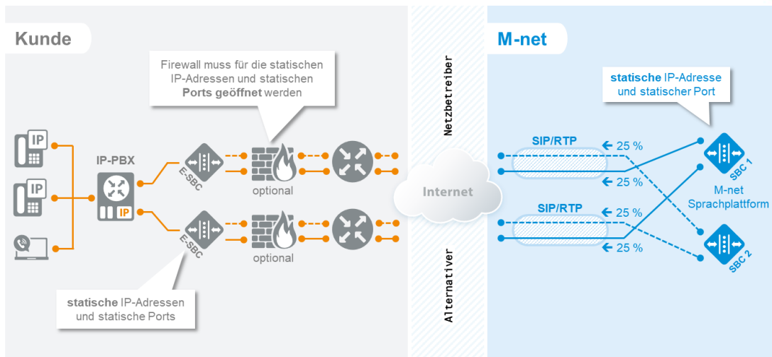
Abbildung 10: Anschaltung einer IP-PBX im SIP-Trunk Static Mode mit Redundanz und Loadbalancing bei Vollvermaschung über Internet-Access durch Alternativanbieter
