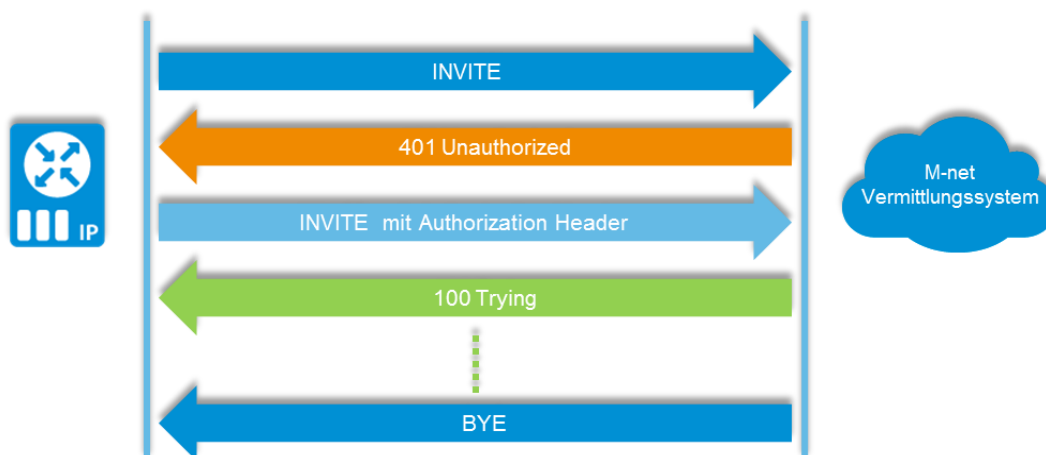
Abbildung 13: Beispiel Gesprächsauthentifizierung
